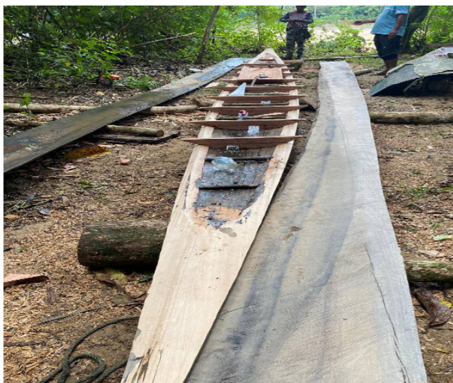
Gambaran Awal Perahu Jalur dengan Bahagian Lunas di Tengah Sebelum Papan Timbal Kiri dan Kanan di Pasang
